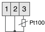
Zapojení Pt100
