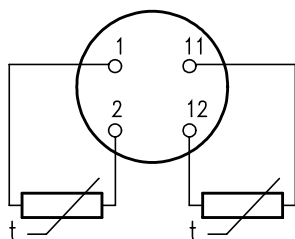
s dvojitým měřicím odporem ve dvou vodičovém zapojení (2 x Pt 100/B/2)
