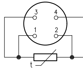
s jednoduchým měřicím odporem ve čtyřvodičovém zapojení (Pt 100/ /4)
