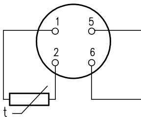
s jednoduchým měřicím odporem v zapojení s pomocnou smyčkou (Pt 100/B/4)
