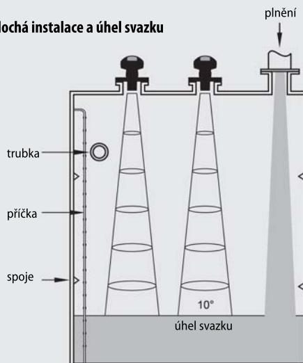
Instalace sondy SISTRANS LU
